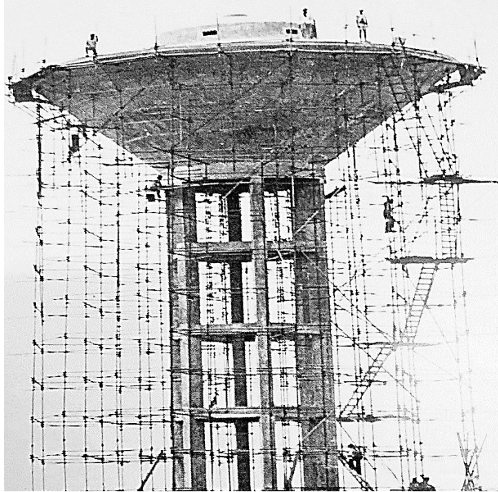
Photo N°2: Le nouveau château d'eau de Katiola
